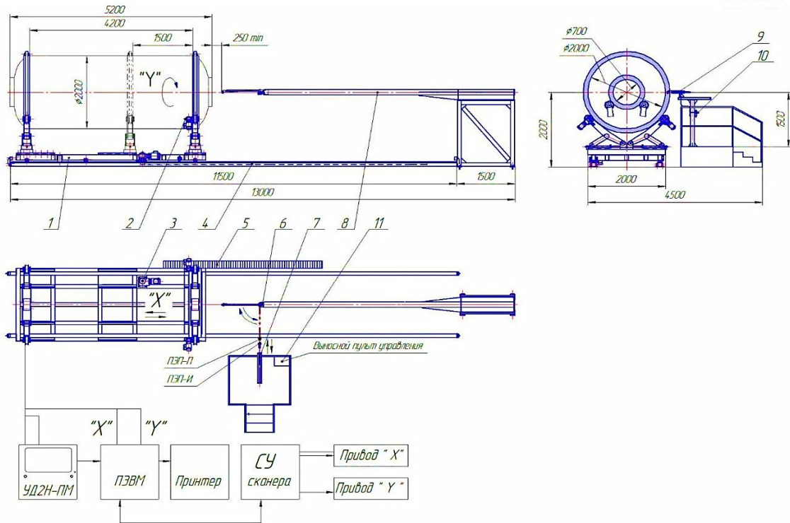
Компоновочная схема установки ASIQ-1
